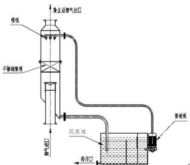
图 4.2.1-3 水膜除尘器原理与结构示意图
