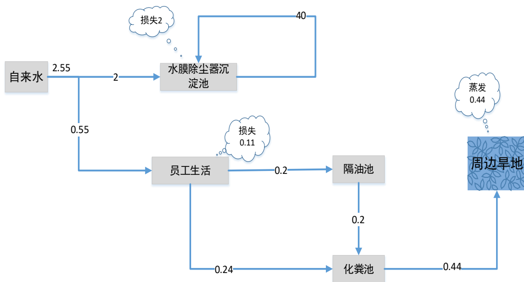
图 2-1 项目运营期水平衡图 单位：m 3 /d
