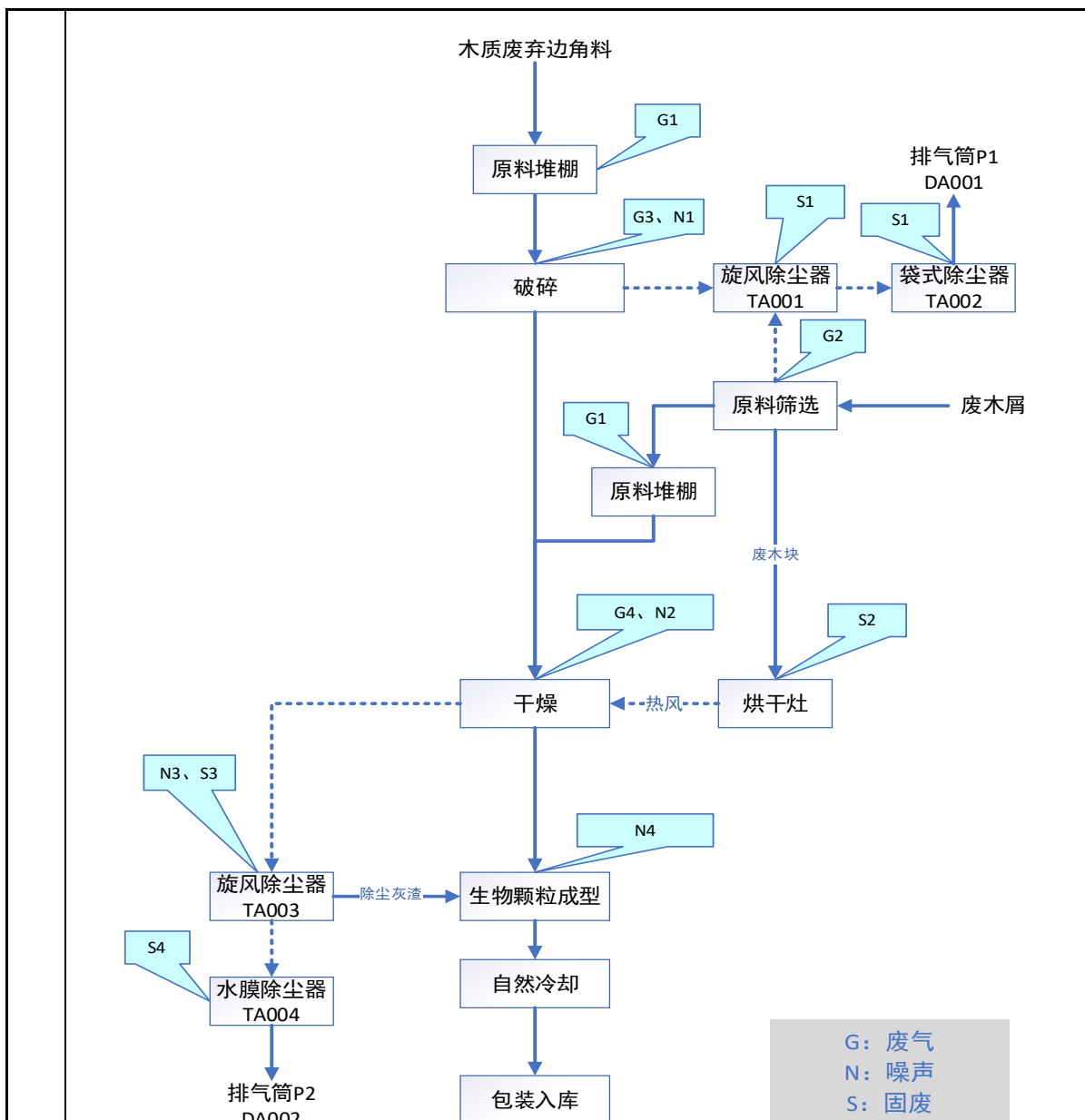
图 2-2 项目生产工艺及产污节点图
