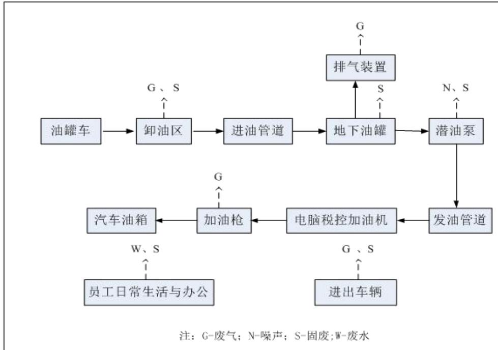
图 2-1 加油站工艺流程和产污节点图
